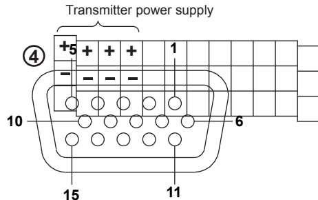
D-Sub 15-pin receptacle
