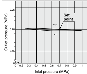
AWD30
