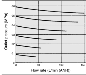
AWD20 Rc 1/4
