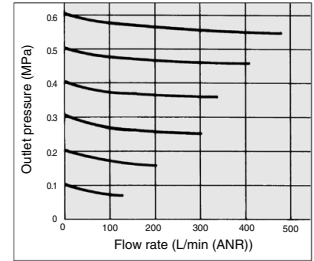
AWD40 Rc 1/2
