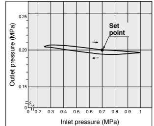
AWD40
