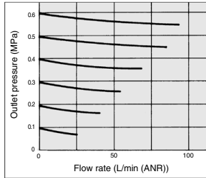
AWD20 Rc 1/4
