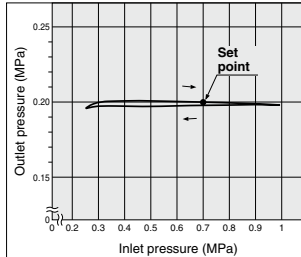
AWD20
