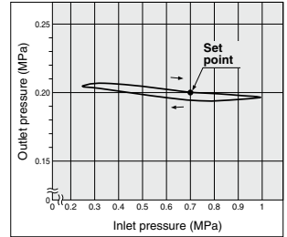
AWD40
