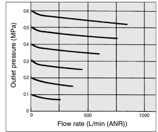
AWD40 Rc 1/2
