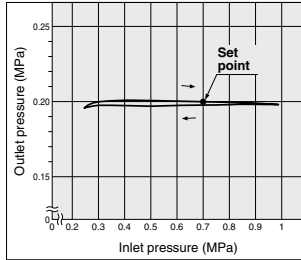
AWD20
