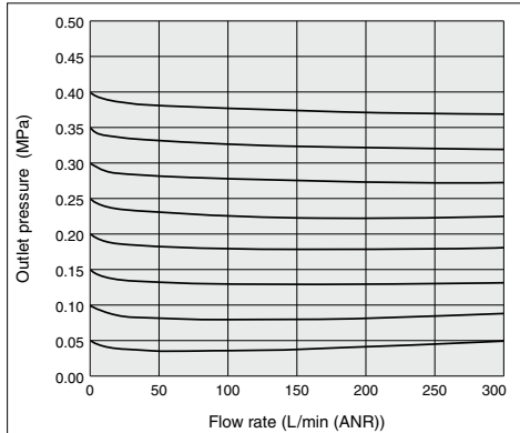
ARP20(K) Rc 1/4
