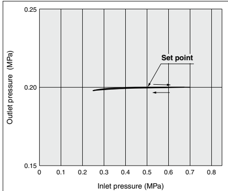
ARP30(K)
