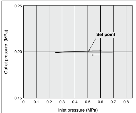
ARP40(K)
