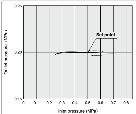
ARP20(K)
