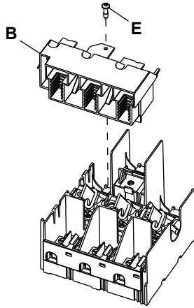
Figure / Figura / Figure 3 : Arc Shield/Suppressor Installation / Instalación del blindaje/supresor de arco / Installation du blindage/suppresseur d'arc
