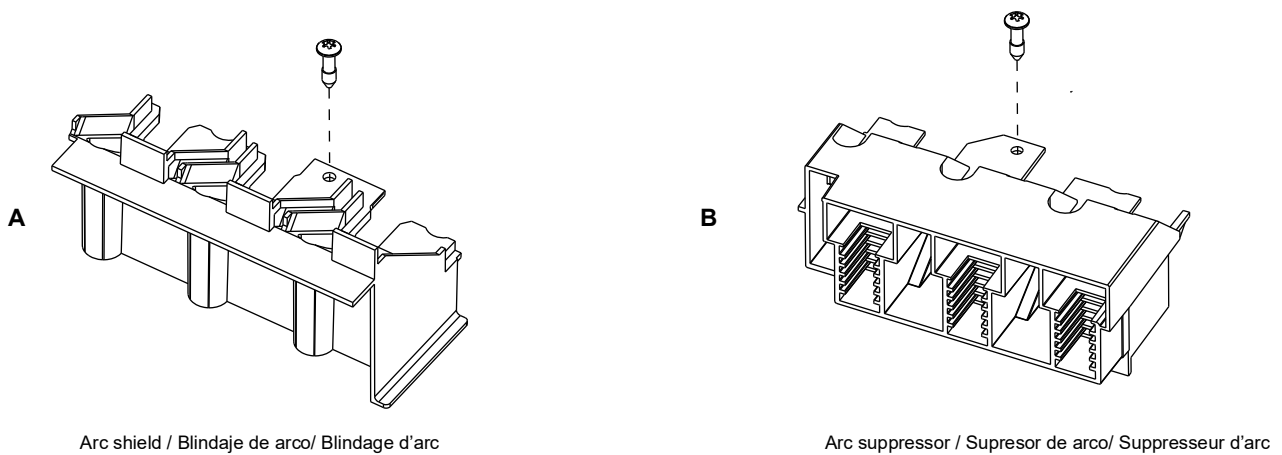
Figure / Figura / Figure 1 : Arc Shield and Arc Suppressor Housing / Blindaje de arco y caja de supresor de arco / Blindage d'arc et boîtier supresseur d'arc
