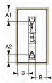
1P
