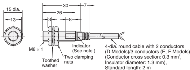
Fig. 4 : E2E-X2D□-N E2E-X1R5E□/F□
