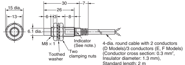
Fig. 5 : E2E-X4MD□ E2E-X2ME□/F□
