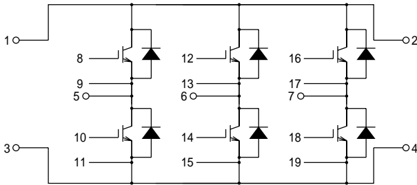
回路図 CIRCUIT
