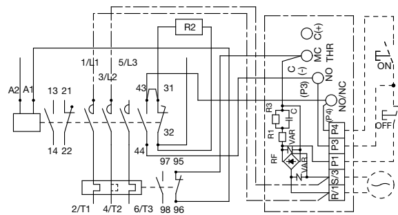
MSO-T21DL(KP) Actual Wiring Diagram
