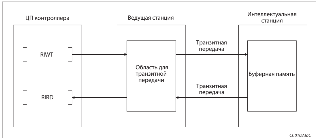
Рис. 1-7: Транзитная передача данных с интеллектуальной станцией
