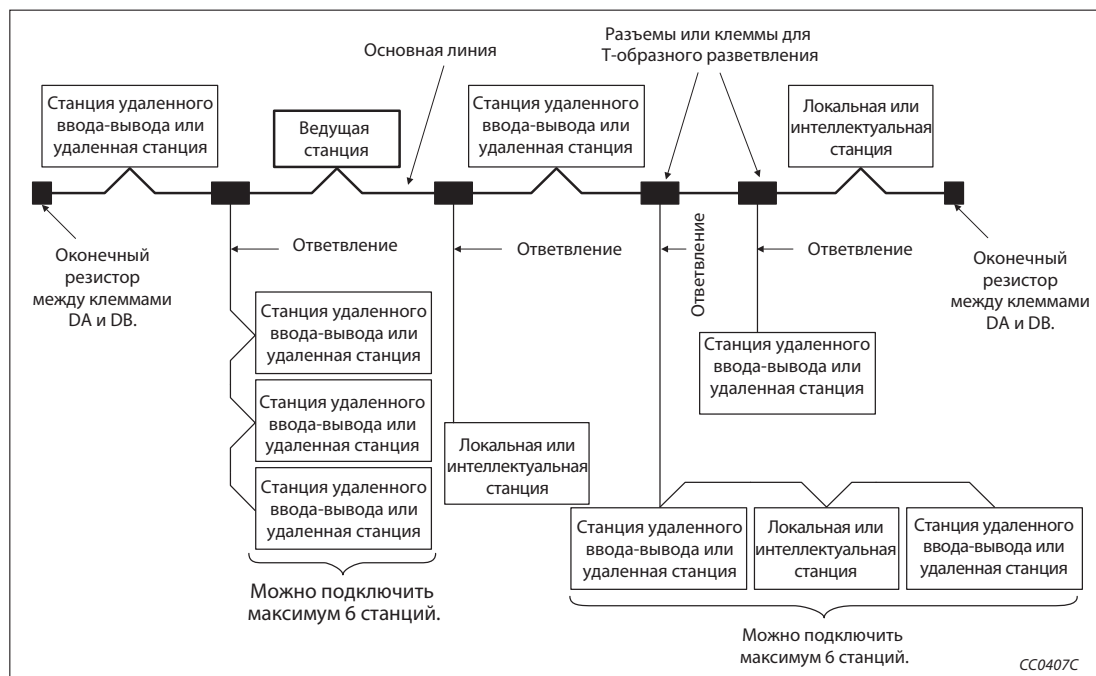
Рис. 7-7: Построение коммуникационной сети с T-образными разветвлениями
