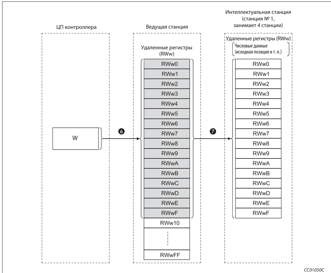
Рис. 4-19: Передача данных в удаленные регистры
