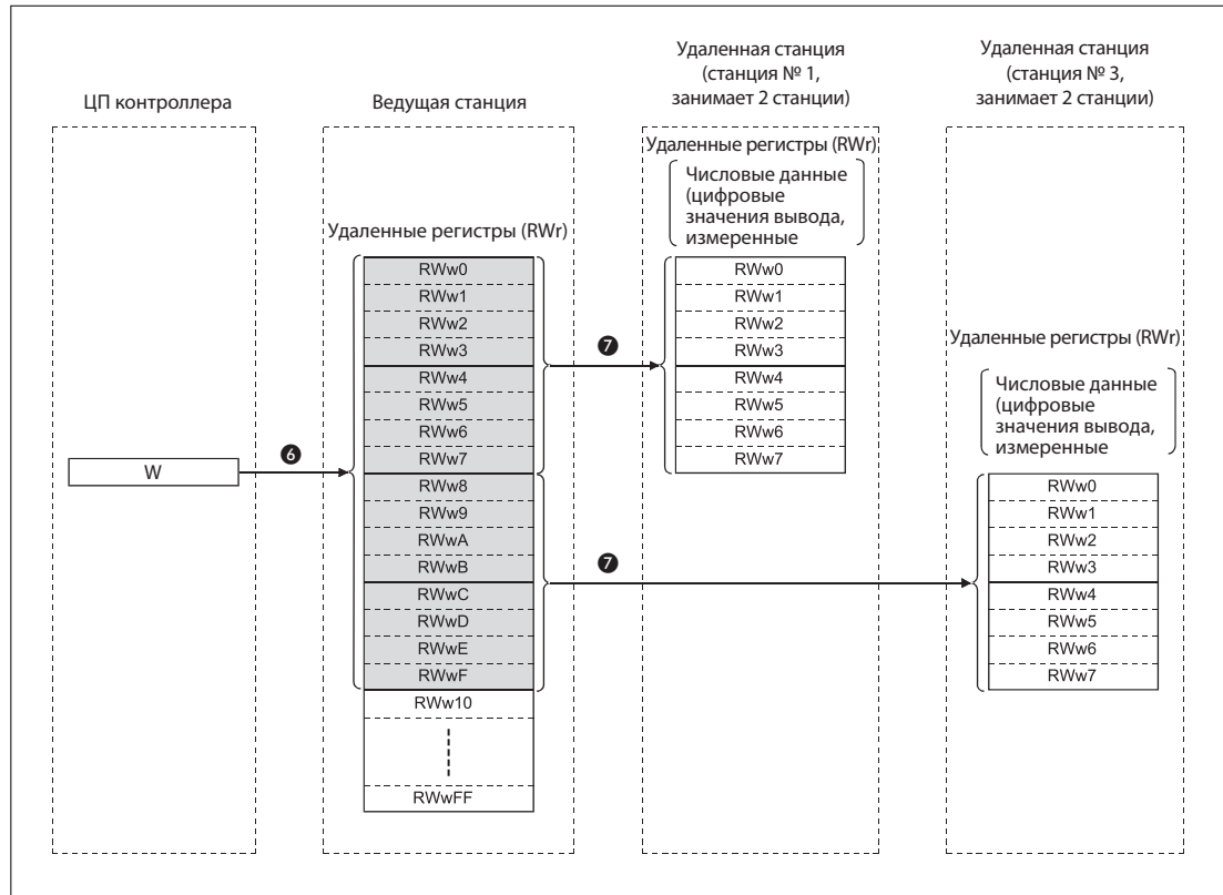
Рис. 4-7: Передача данных в удаленные регистры (RWw)
