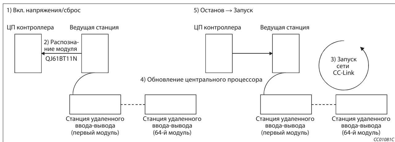
Рис. 4-4: Конфигурация системы
