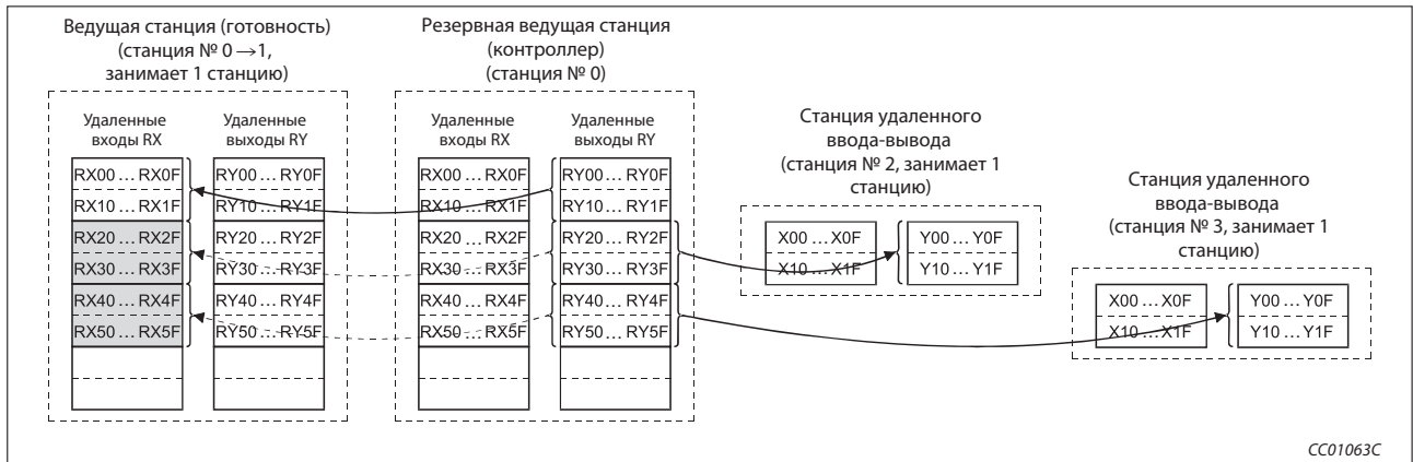
Рис. 4-34: Вывод из резервной ведущей станции
