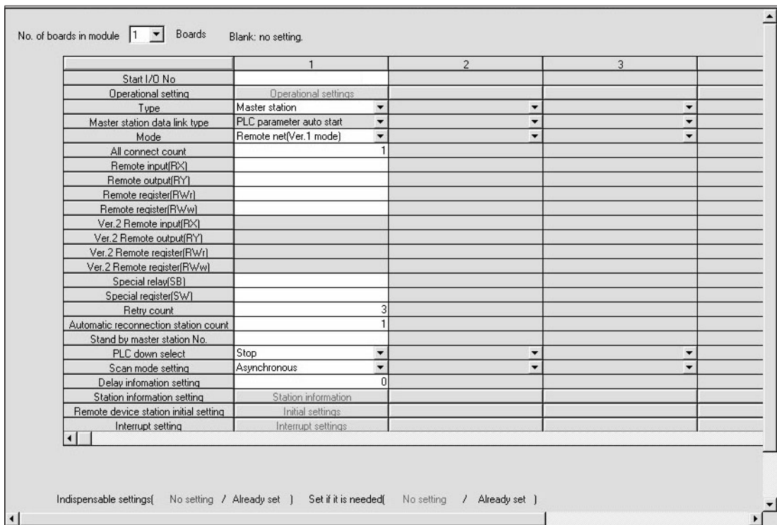
Рис. 11-3: Настройка сетевых параметров в GX IEC Developer
