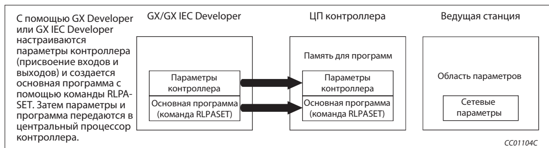
Рис. 6-4: Передача параметров в центральный процессор контроллера
