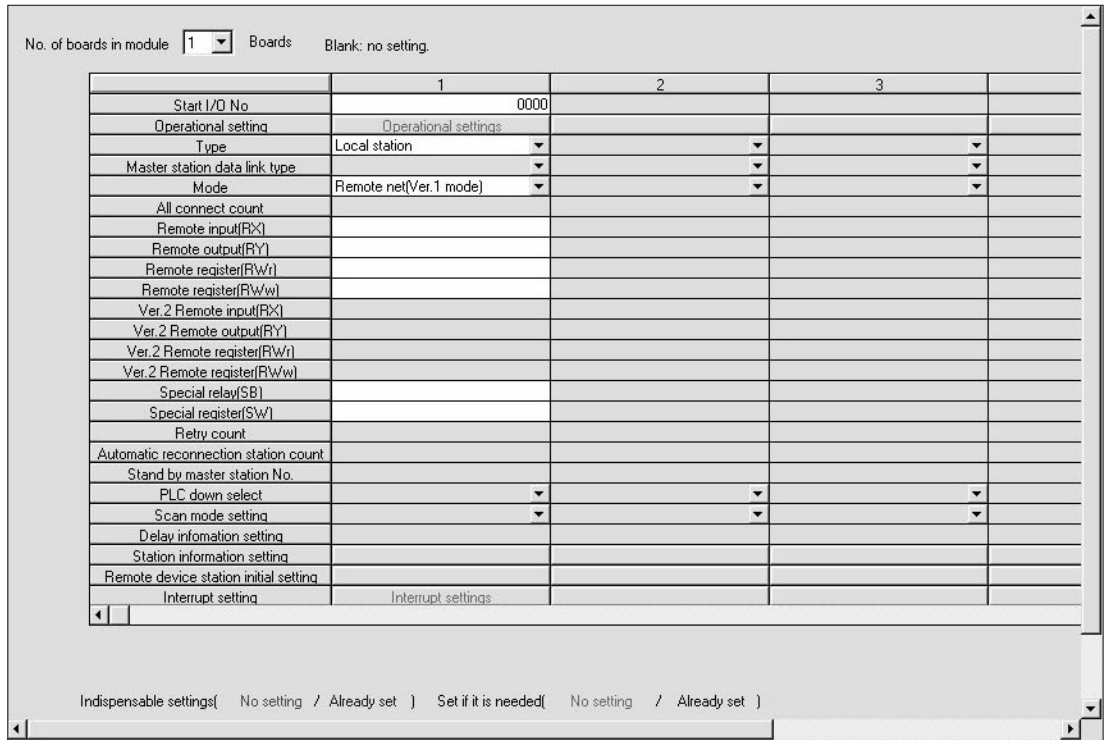
Рис. 11-18: Настройка сетевых параметров в GX IEC Developer
