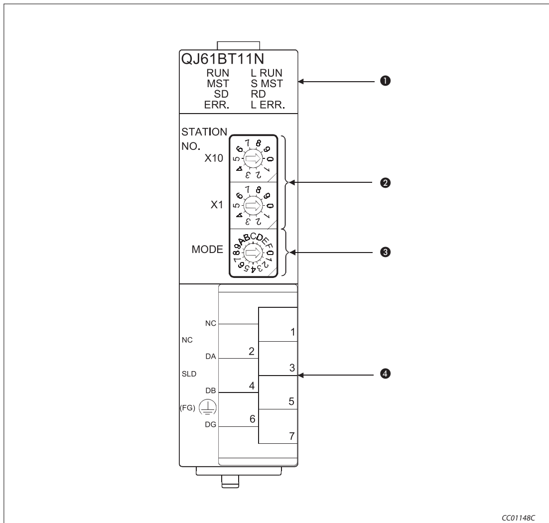
Рис. 7-3: Элементы управления ведущего и локальных модулей CC-Link
