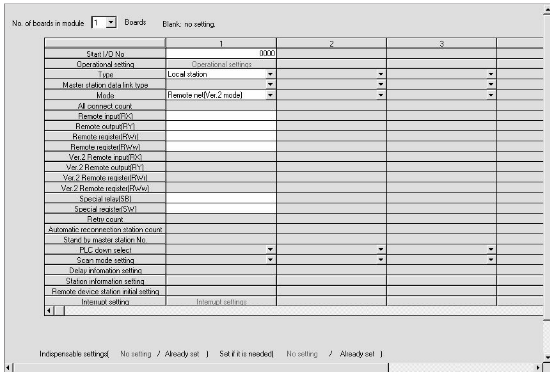
Рис. 11-20: Настройка сетевых параметров в GX IEC Developer
