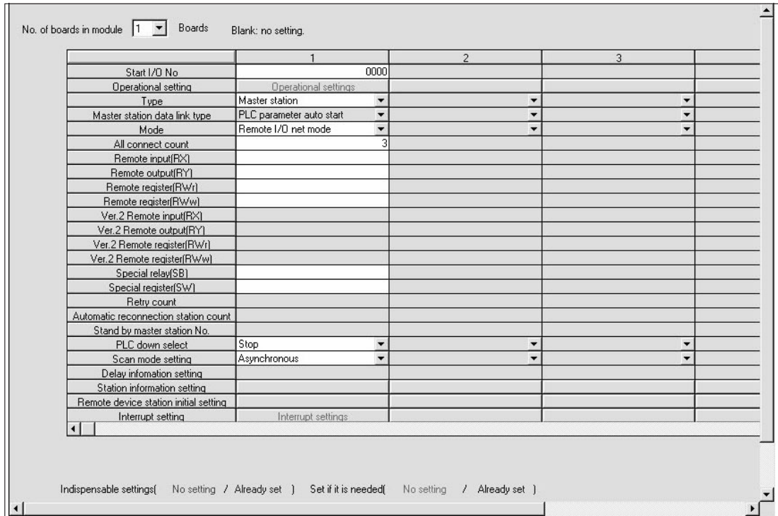
Рис. 9-4: Настройка сетевых параметров в GX IEC Developer
