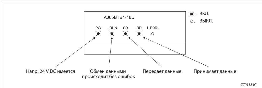
Рис. 9-9: Светодиодные индикаторы на станциях удаленного ввода-вывода
