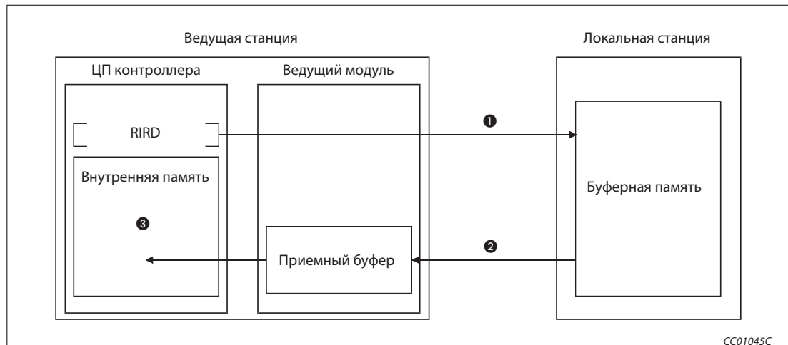
Рис. 4-15: Считывание данных командой RIRD
