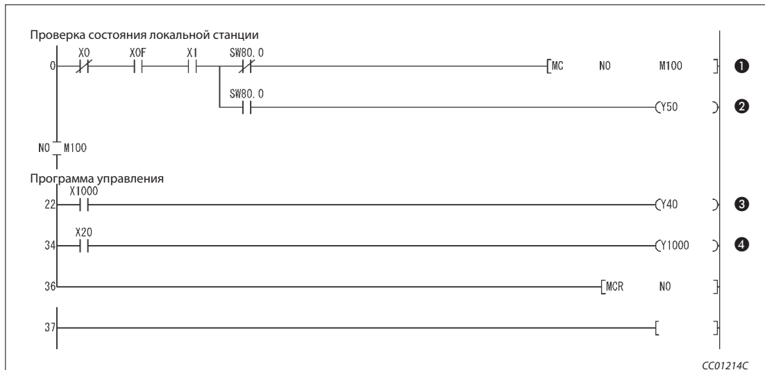
Рис. 11-9: Основная программа ведущей станции
