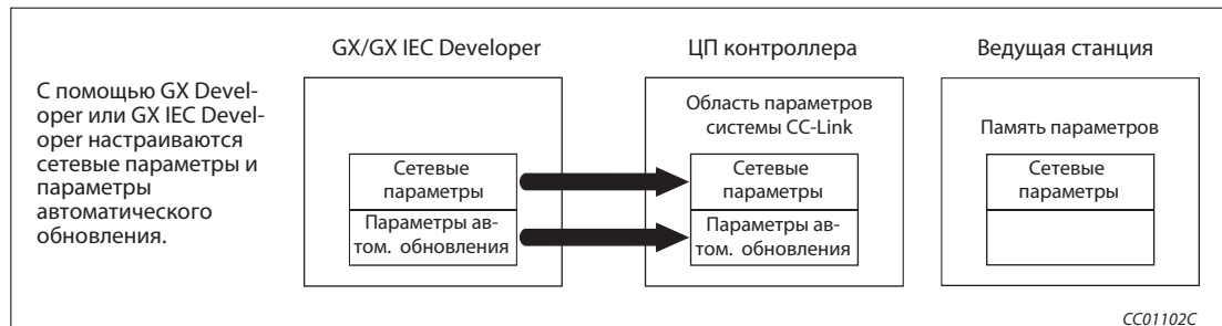
Рис. 6-3: Передача параметров в центральный процессор контроллера
