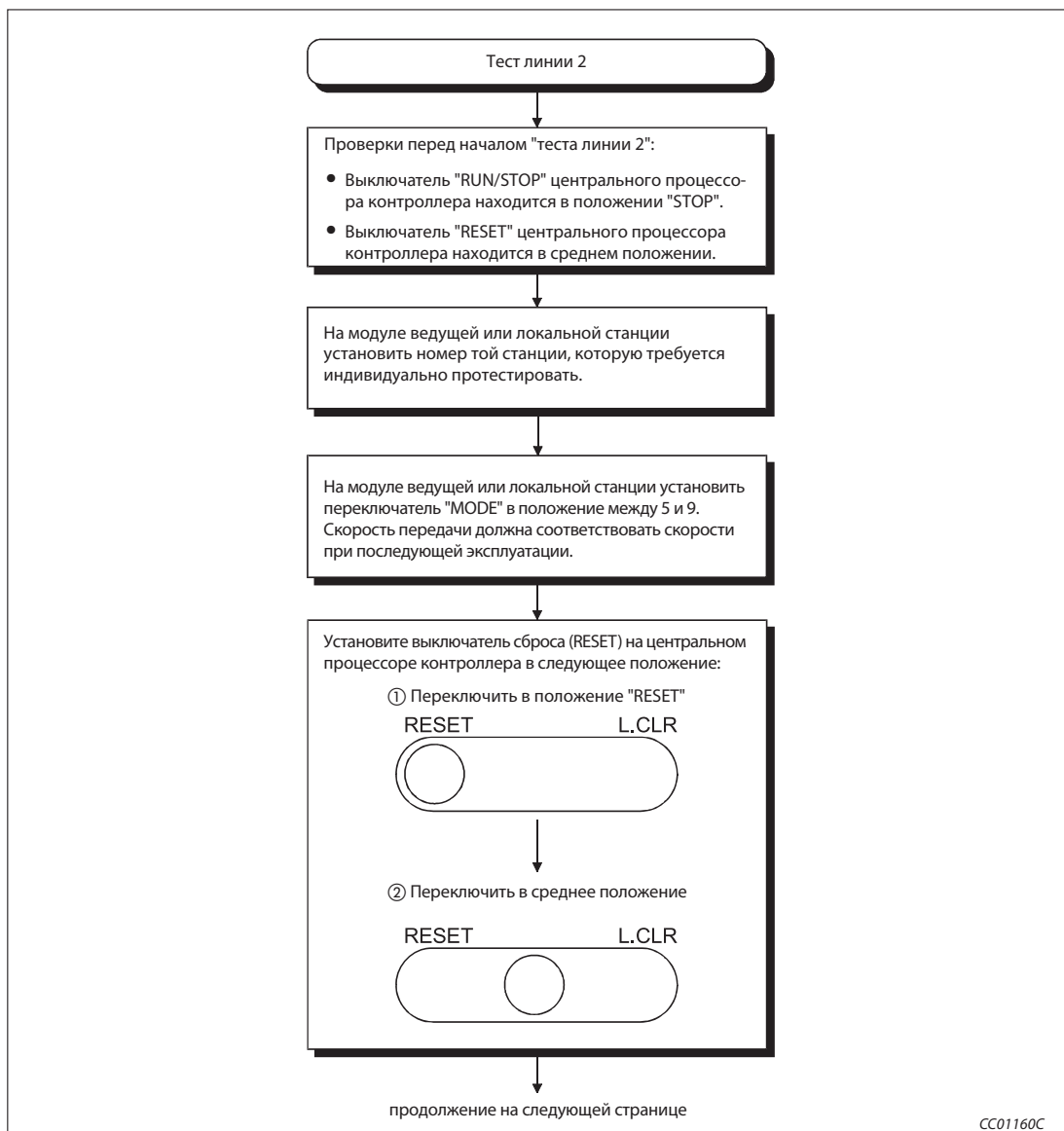
Рис. 7-11: Порядок действий для тестирования линии 2 (1)
