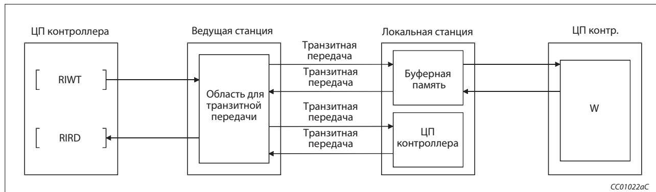
Рис. 1-5: Транзитная передача данных с локальной станцией
