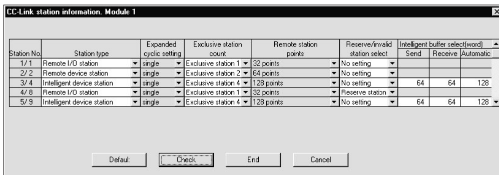
Рис. 6-1: Меню "Информация о станциях CC-Link"
