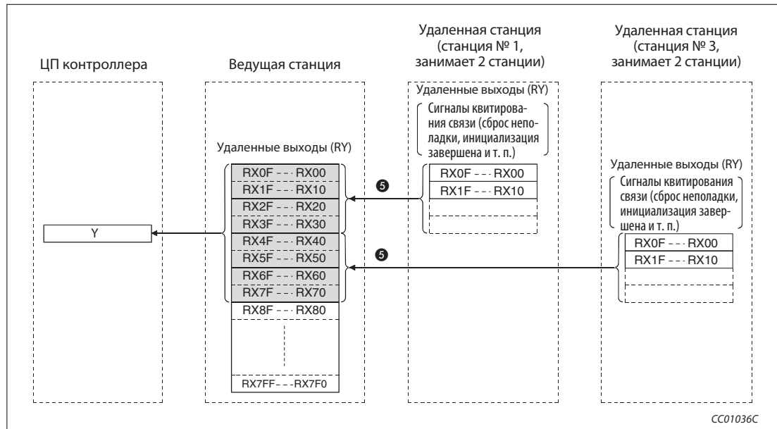
Рис. 4-5: Определение состояний удаленных входов удаленных станций
