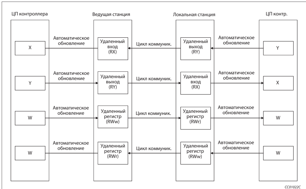
Рис. 1-4: Циклическая передача данных с локальной станцией
