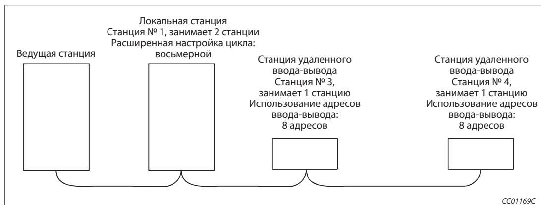
Рис. 8-8: Пример системы для пояснения смещений и используемых адресов
