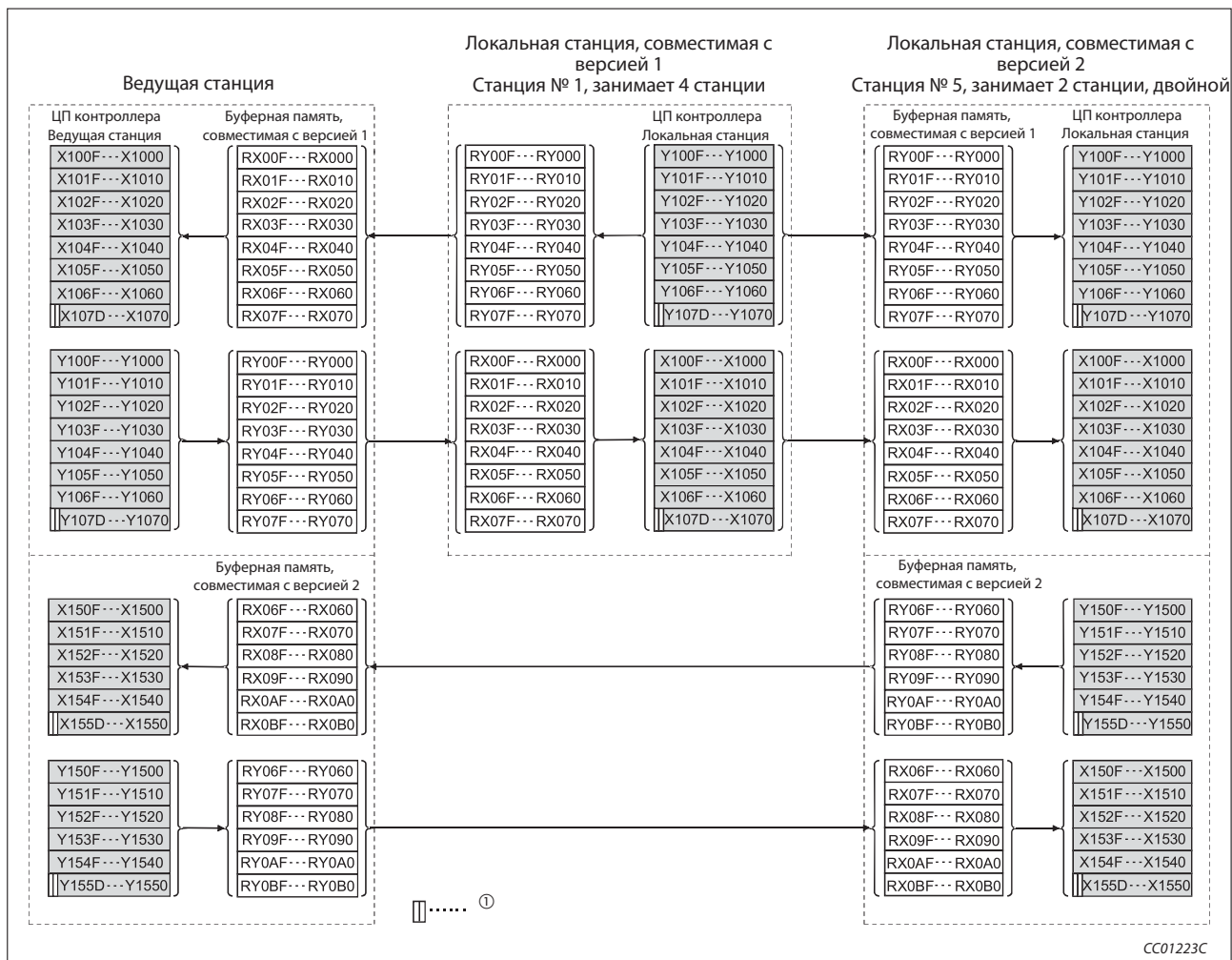
Рис. 11-37: Удаленные входы (RX) и выходы (RY)
