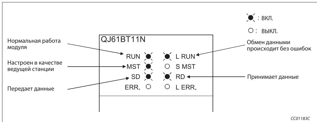
Рис. 9-8: Светодиодные индикаторы на ведущей станции
