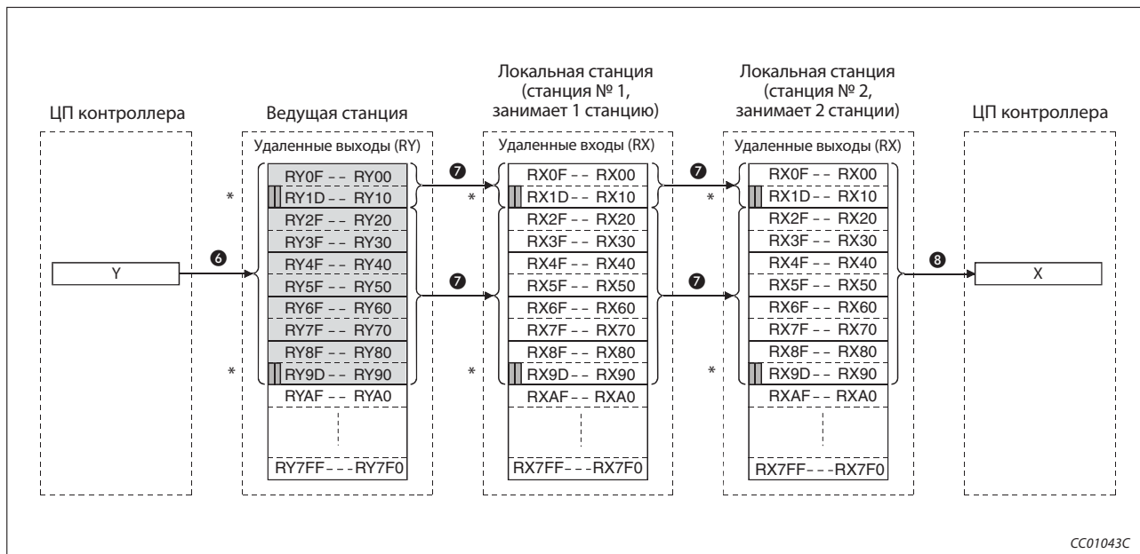
Рис. 4-11: Данные (RY) от локальной к ведущей и другим локальным станциям
