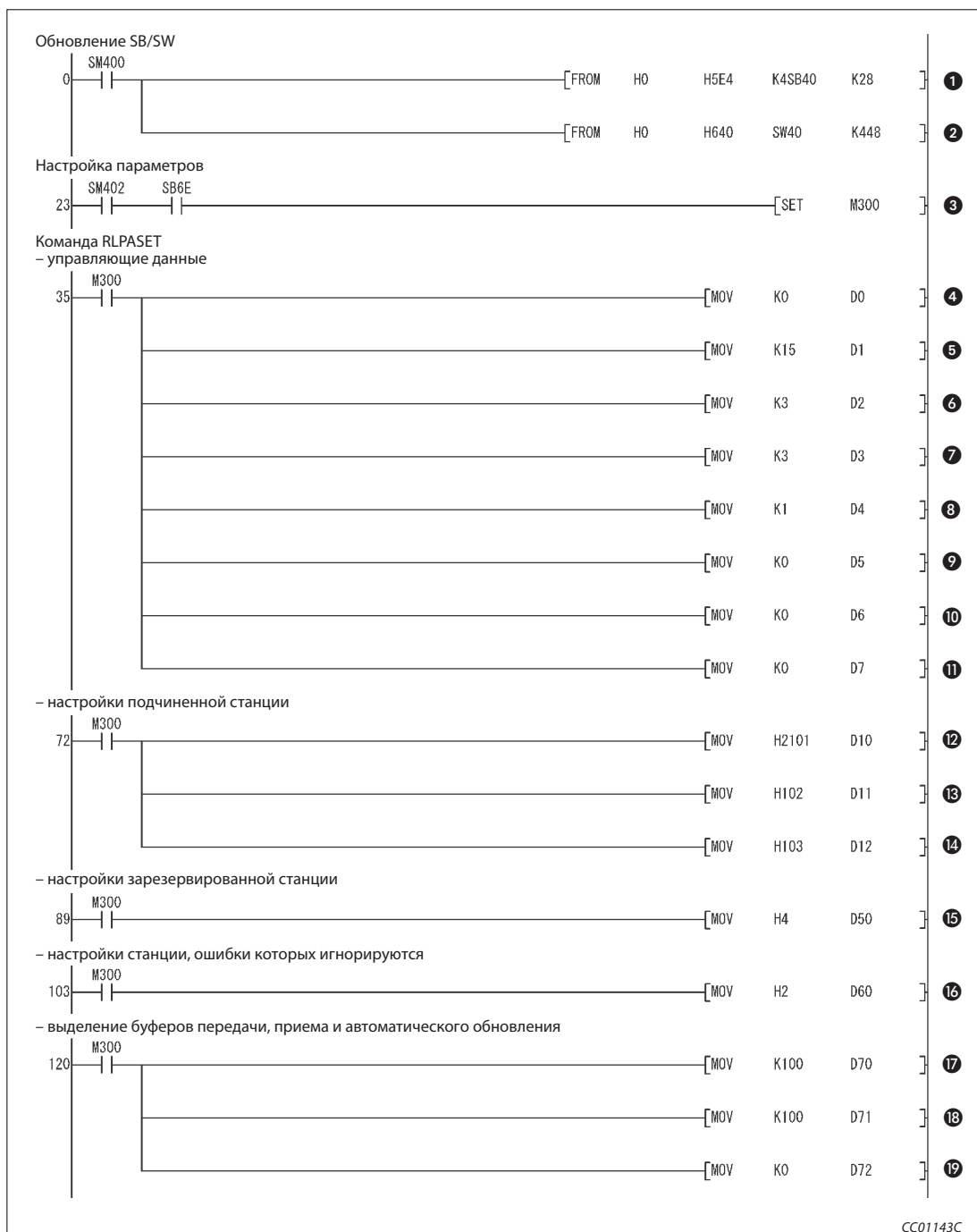
Рис. 6-26: Пример программы (релейно-контактная схема GX Developer) (1)
