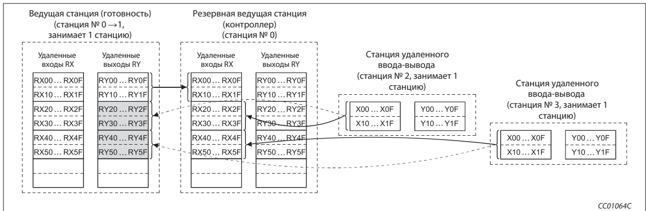
Рис. 4-35: Ввод в резервную ведущую станцию
