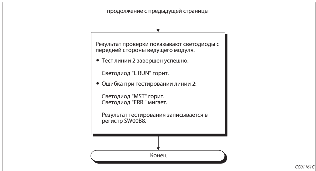
Рис. 7-11: Порядок действий для тестирования линии 2 (2)
