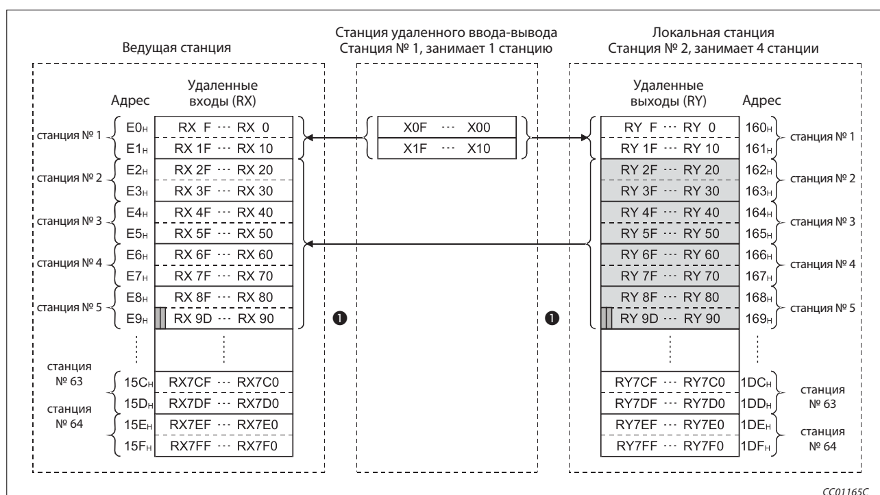
Рис. 8-4: Область буферной памяти для удаленных входов (RX) и выходов (RY)
