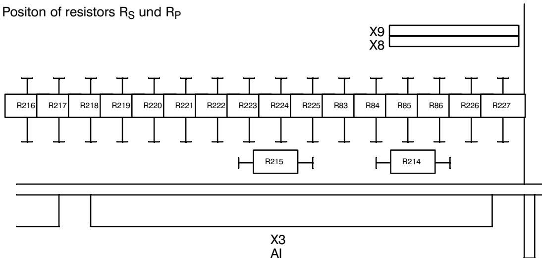
Value of resistors R_S und R_P
