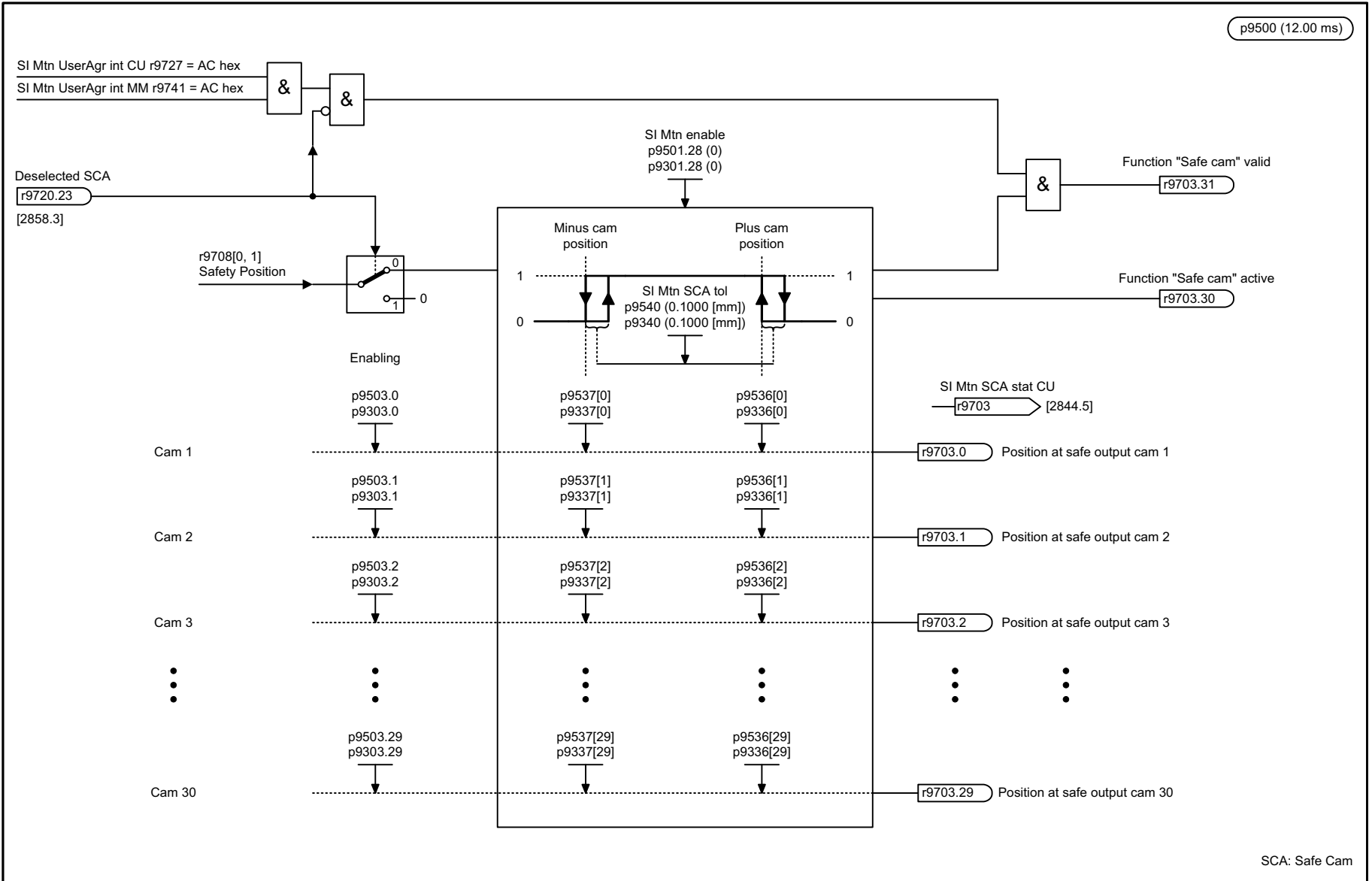
Fig. 3-140 2826 – SCA (Safe Cam)
