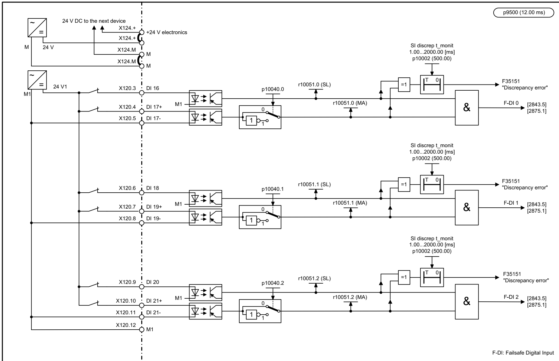
Fig. 3-134 2870 - CU310-2 (F-DI 0 ... F-DI 2)
