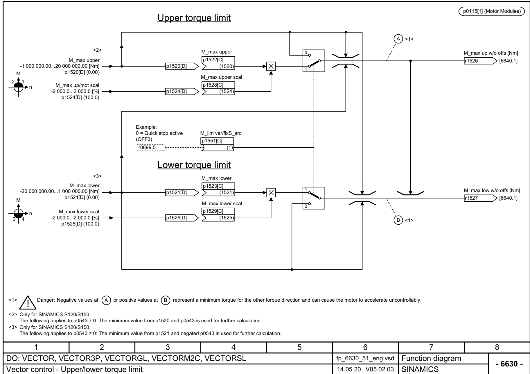
Fig. 3-248 6630 – Upper/lower torque limit
