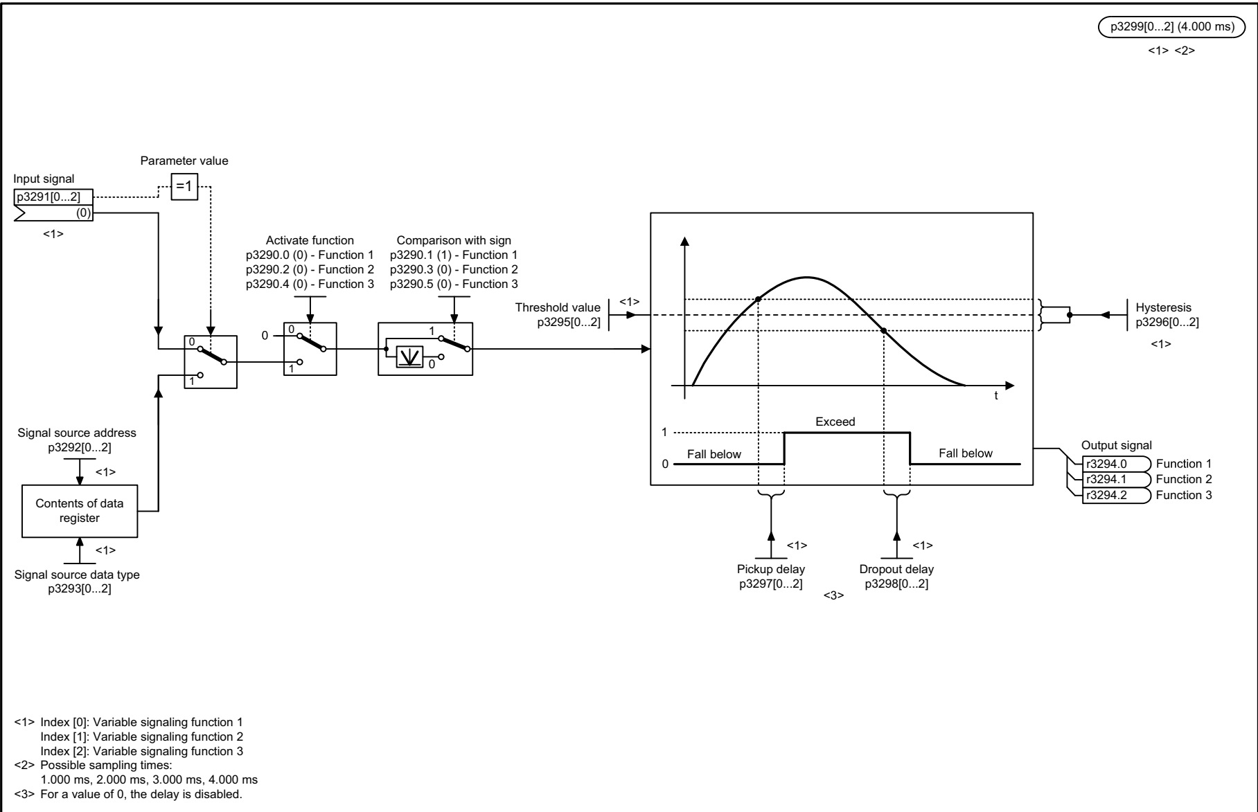
Fig. 3-219 5301 – Variable message function 1, 2, 3
