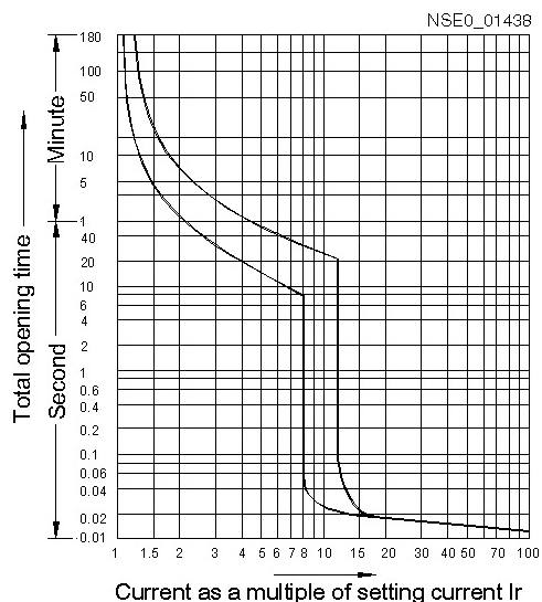
(22) Curvas características do ETU (disparador eletrônico de sobrecorrente)
