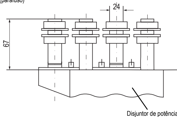
Disjuntor de potência
