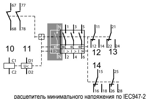
расцепитель минимального напряжения по IEC947-2
