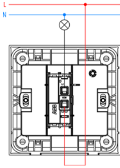
1G 1W switch
