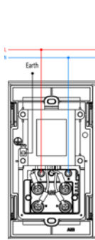
shaver socket
