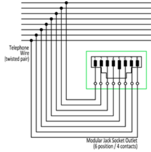
1G / 2G data outlet
