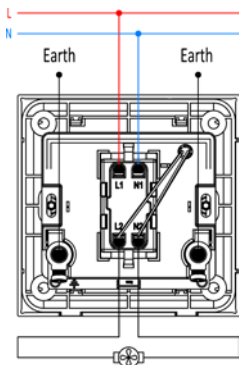
1G 1W DP switch
