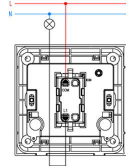
1G 1W 20 AX switch
