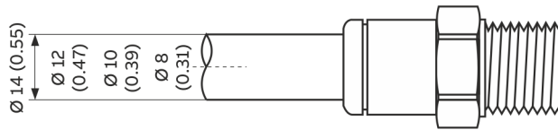
Legris hose adapter (pair)
